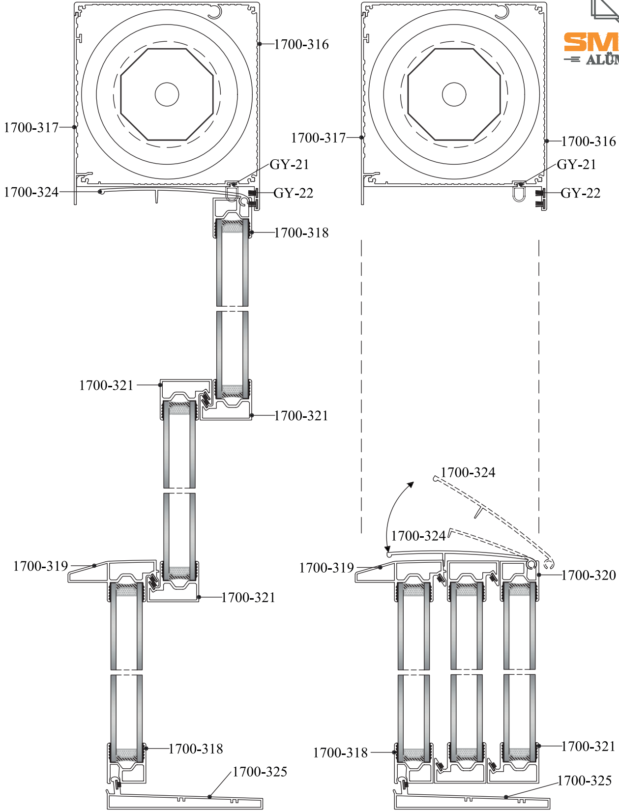
C-C KESİTİ
